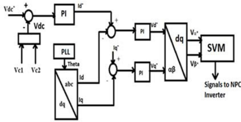
Fig 4. VOC PI controller
