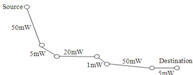
Fig. 3. MINPOW diagram
