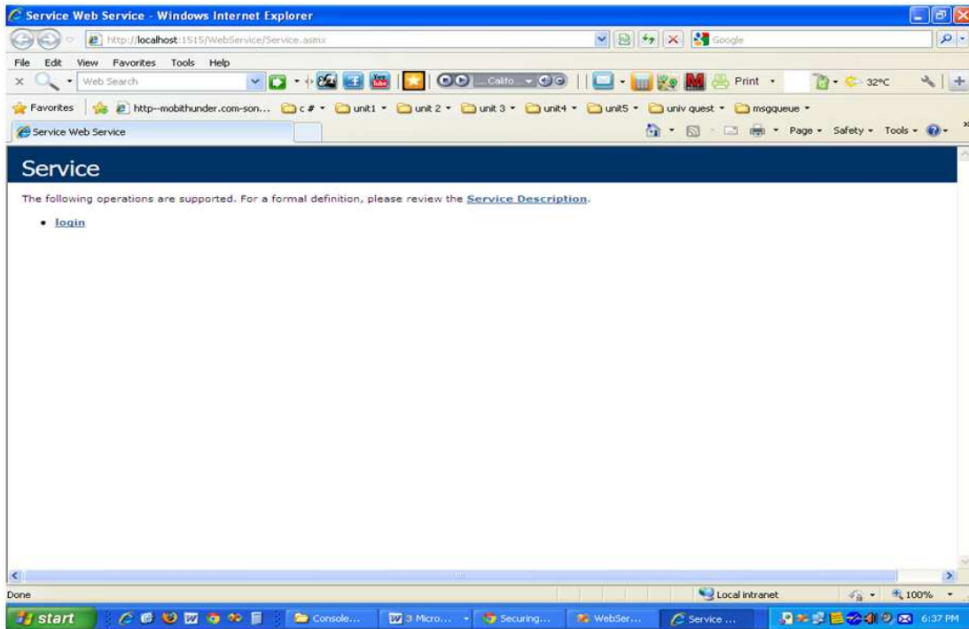
Fig. 5. login service
